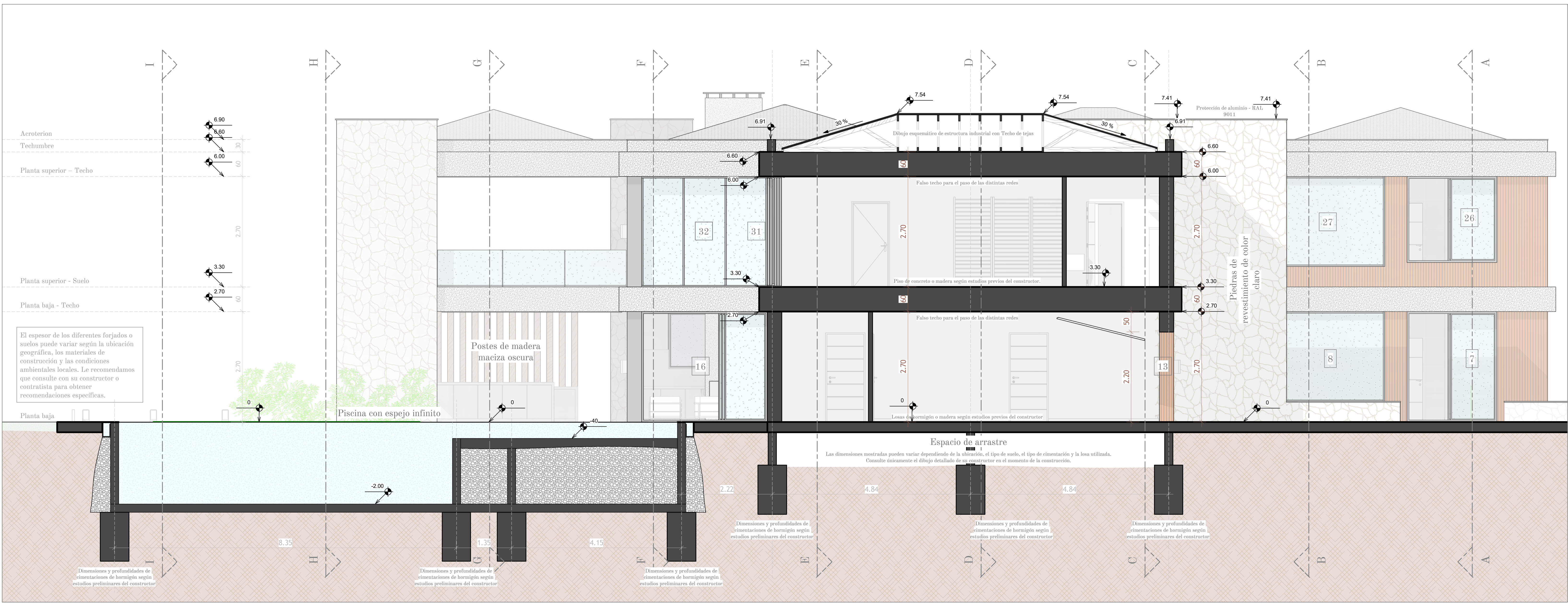
SECCION M-M
