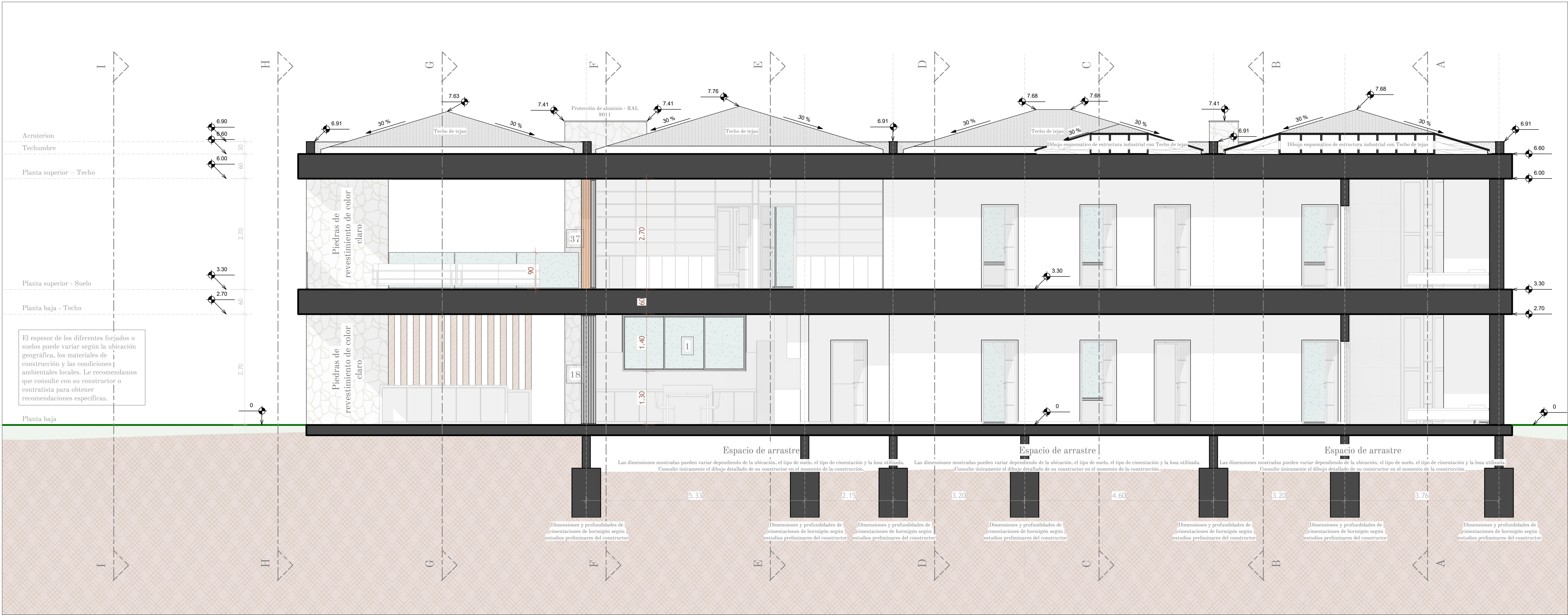
SECCION K-K
