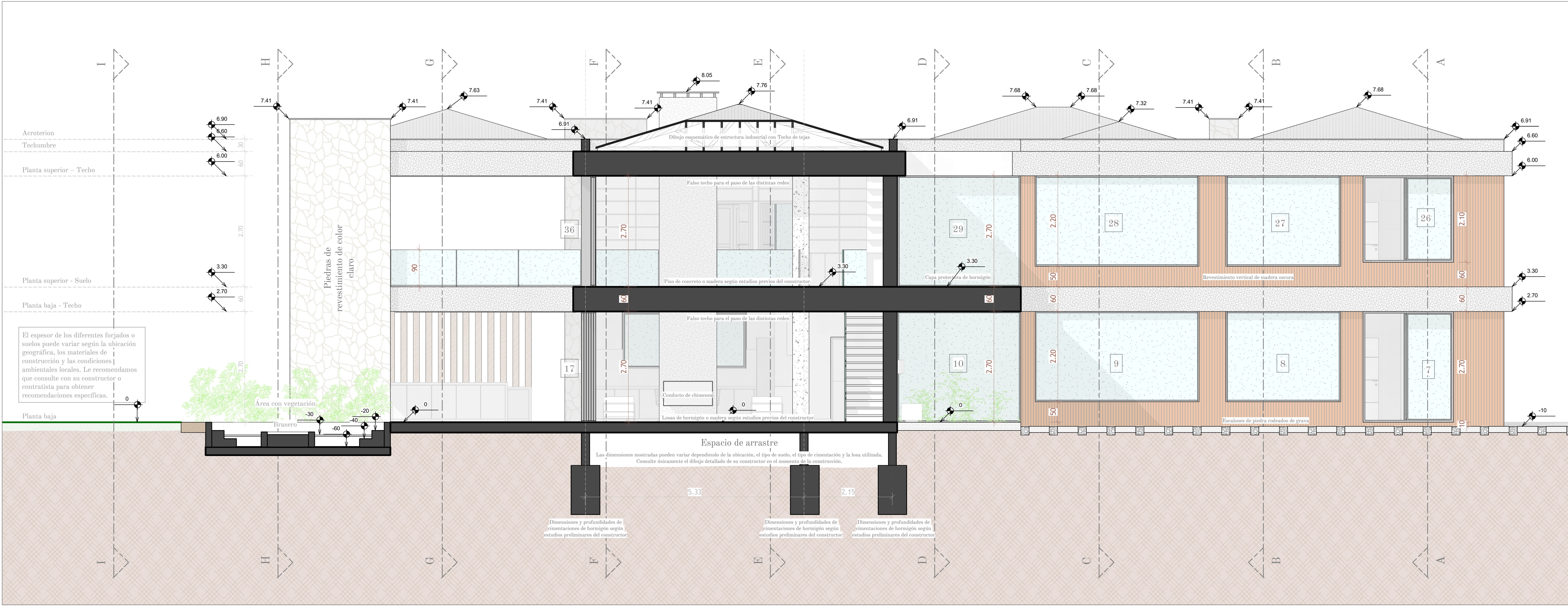
SECCION L-L
