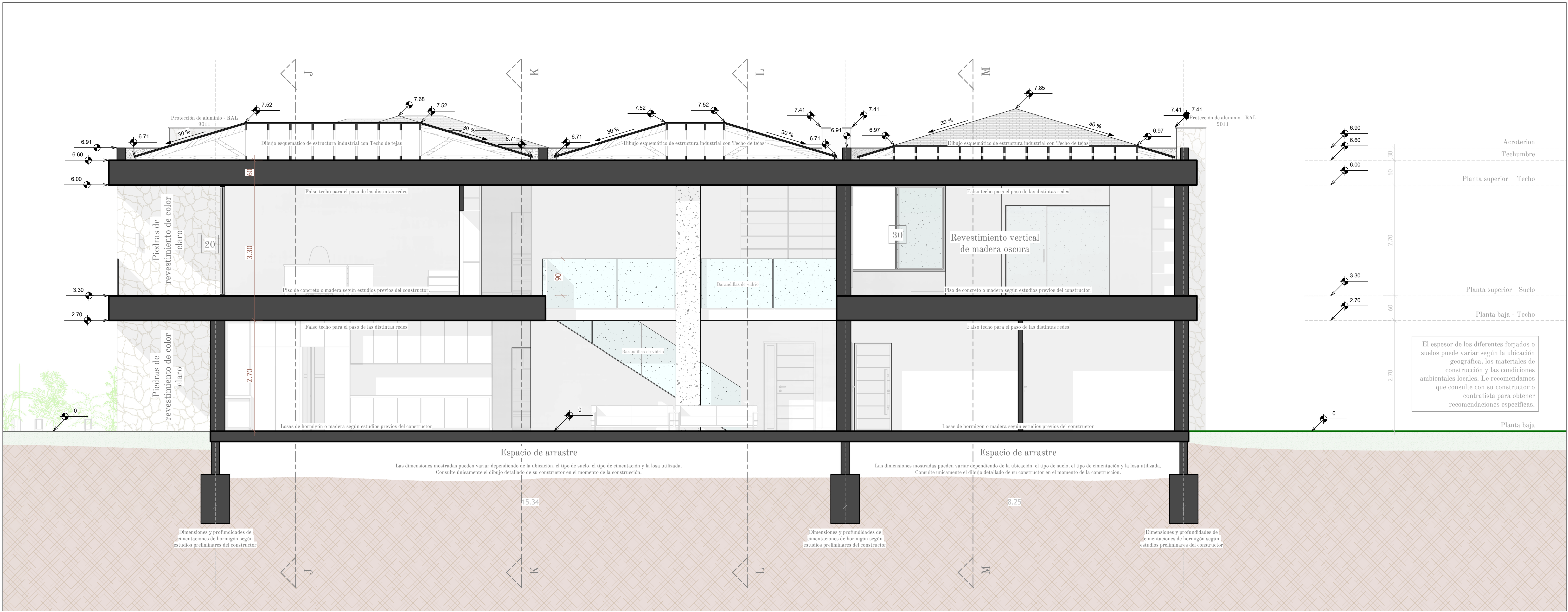
SECCION E-E
